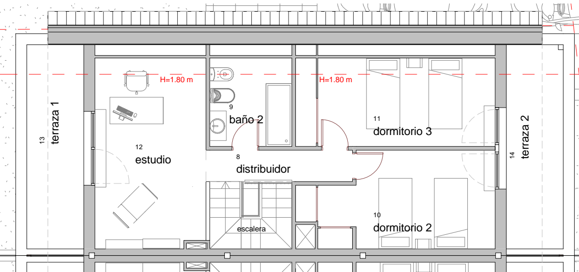
LV04_P. PRIMERA VIVIENDA PR4
