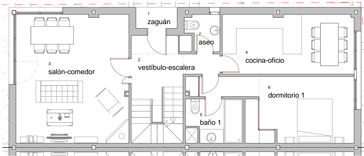
LV04_P. BAJA VIVIENDA PR4
