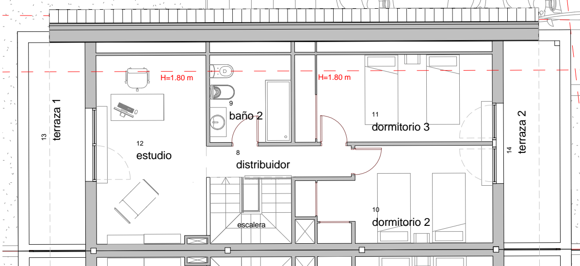
LV02_P. PRIMERA VIVIENDA PR2
