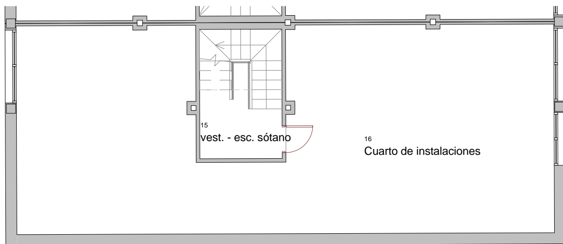
4 LV01_PLANTA SÓTANO VIVIENDA PR1
