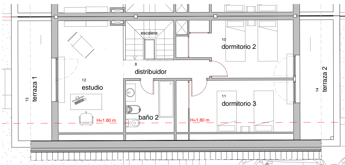
5 LV01_P. PRIMERA VIVIENDA PR1
